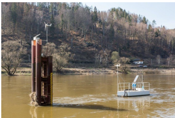
Abb. 8: Dalben und Entnahmebauwerk in der Elbe.
