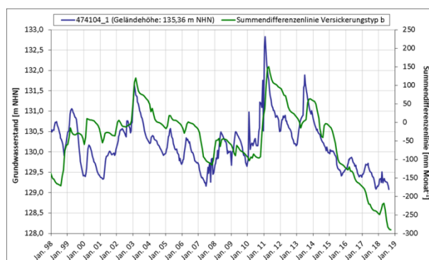
Abb. 3: Grundwasserstand der Messstelle 474104_1 mit Summendifferenzlinie.
